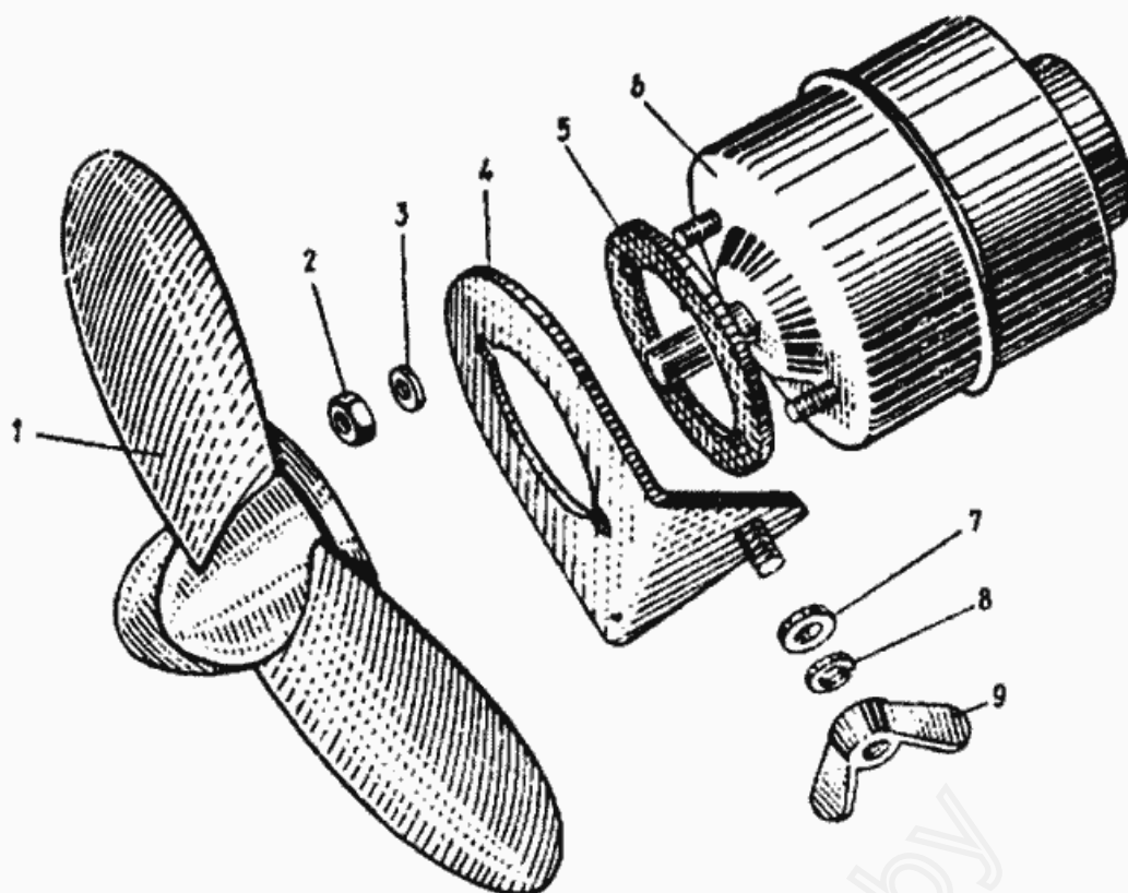
Рис. 69. Вентилятор кабины
